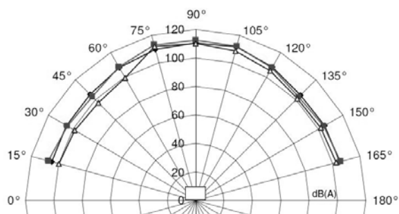
DS 10: Puissance sonore – diagramme horizontale
