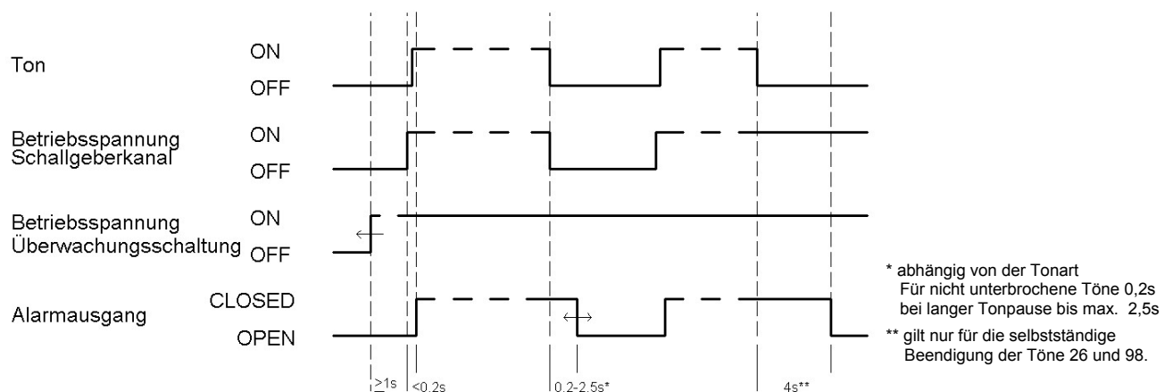
Abb. 7 Funktionszeitdiagramm
