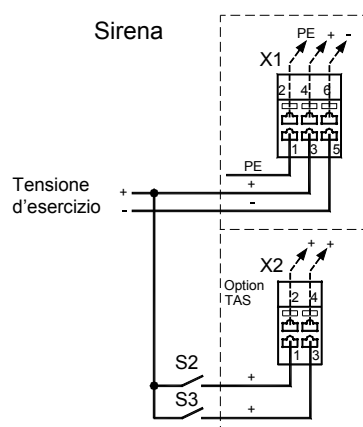
Fig. 10 Assegnazione delle connessioni, opzione TAS
