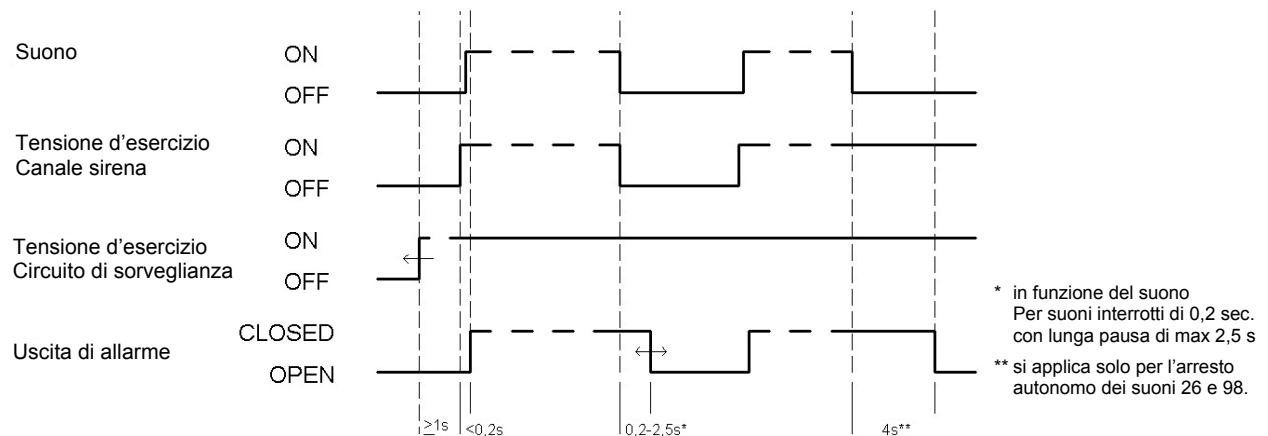
Fig. 7 Diagramma temporale delle funzioni
