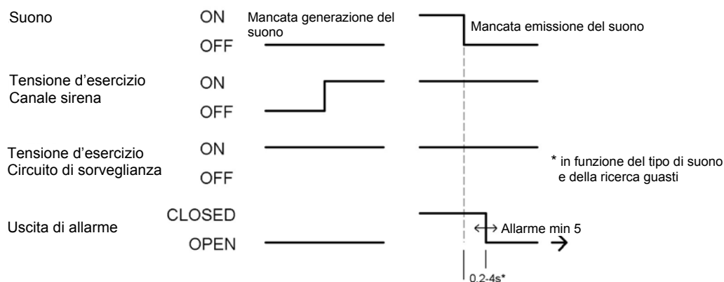
Fig. 8 Diagramma dei tempi funzionali in presenza di guasti
