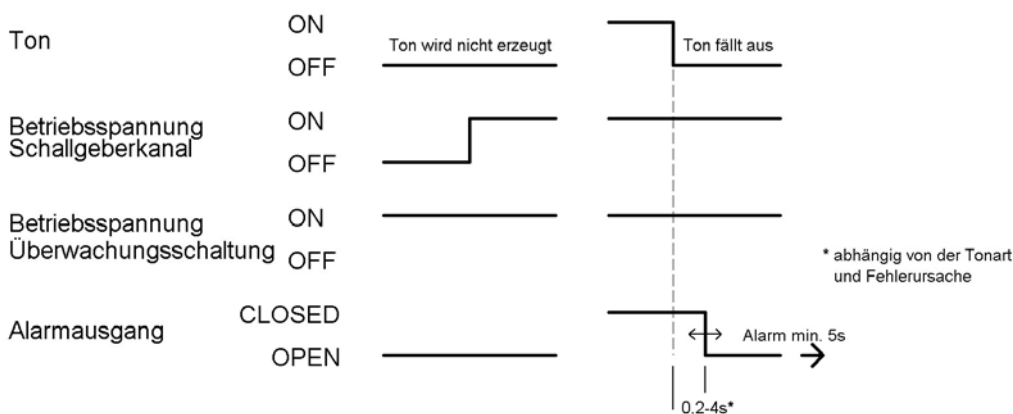
Abb. 9 Funktionszeitdiagramm bei Fehler
