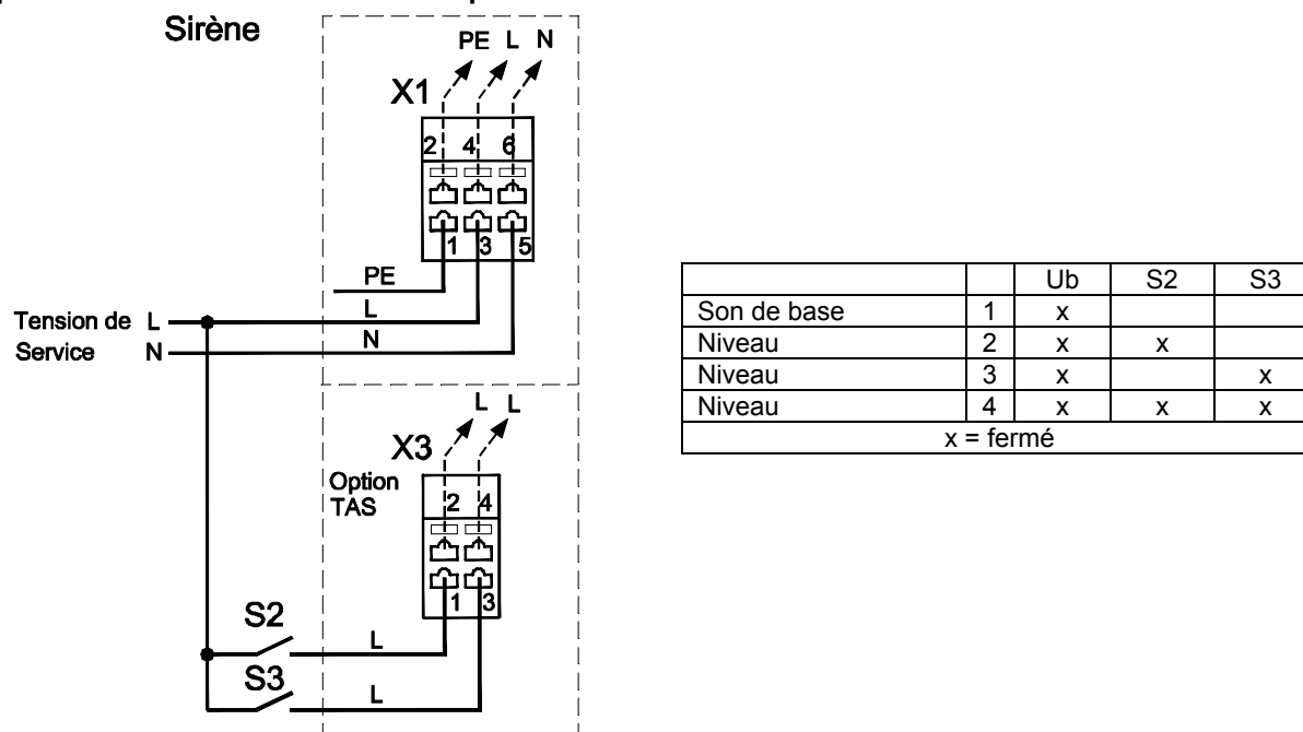
Fig. 11 Affectation des broches avec l'option TAS
