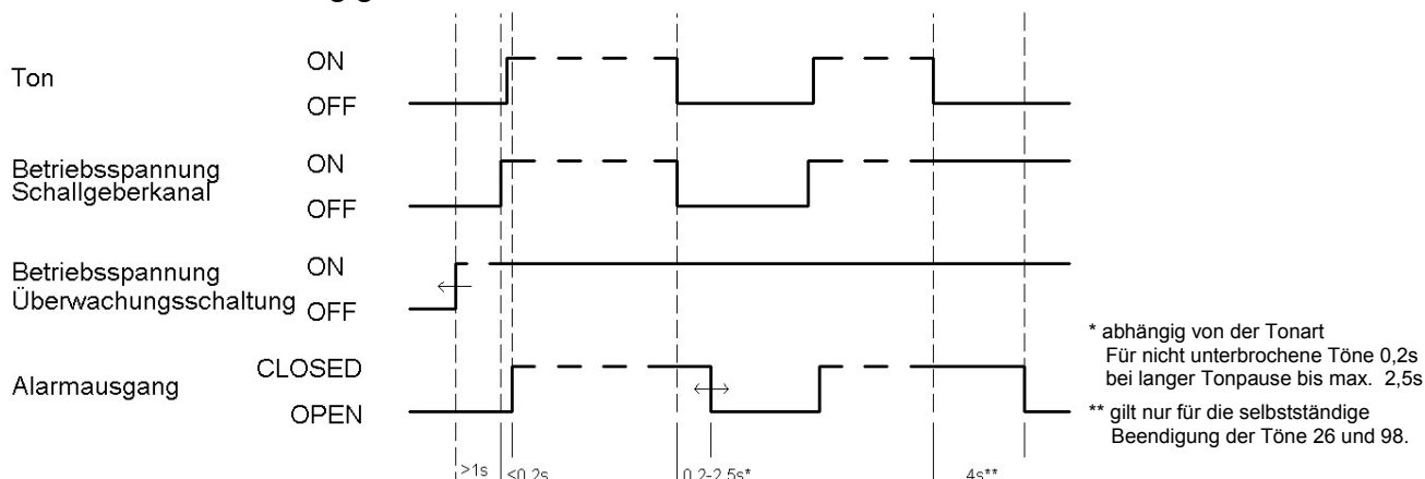
Abb. 8 Funktionszeitdiagramm
