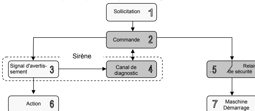
Fig. 5 Signalisation de démarrage
