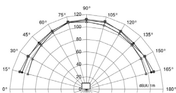
DS 10: Puissance sonore – diagramme vertical
