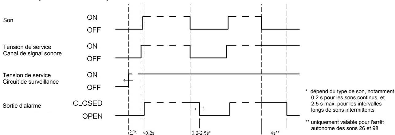
Fig. 8 Diagramme temporel des fonctions
