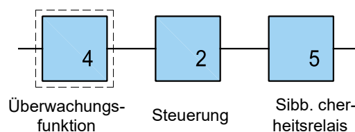
Abb. 8 Sicherheitsrelevantes Blockdiagramm
