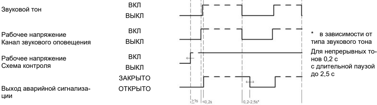
Рис. 9 Временная диаграмма функции для бесперебойного функционирования
