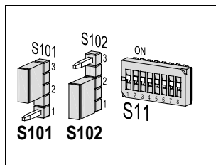
Переключатели на плате драйвера:
